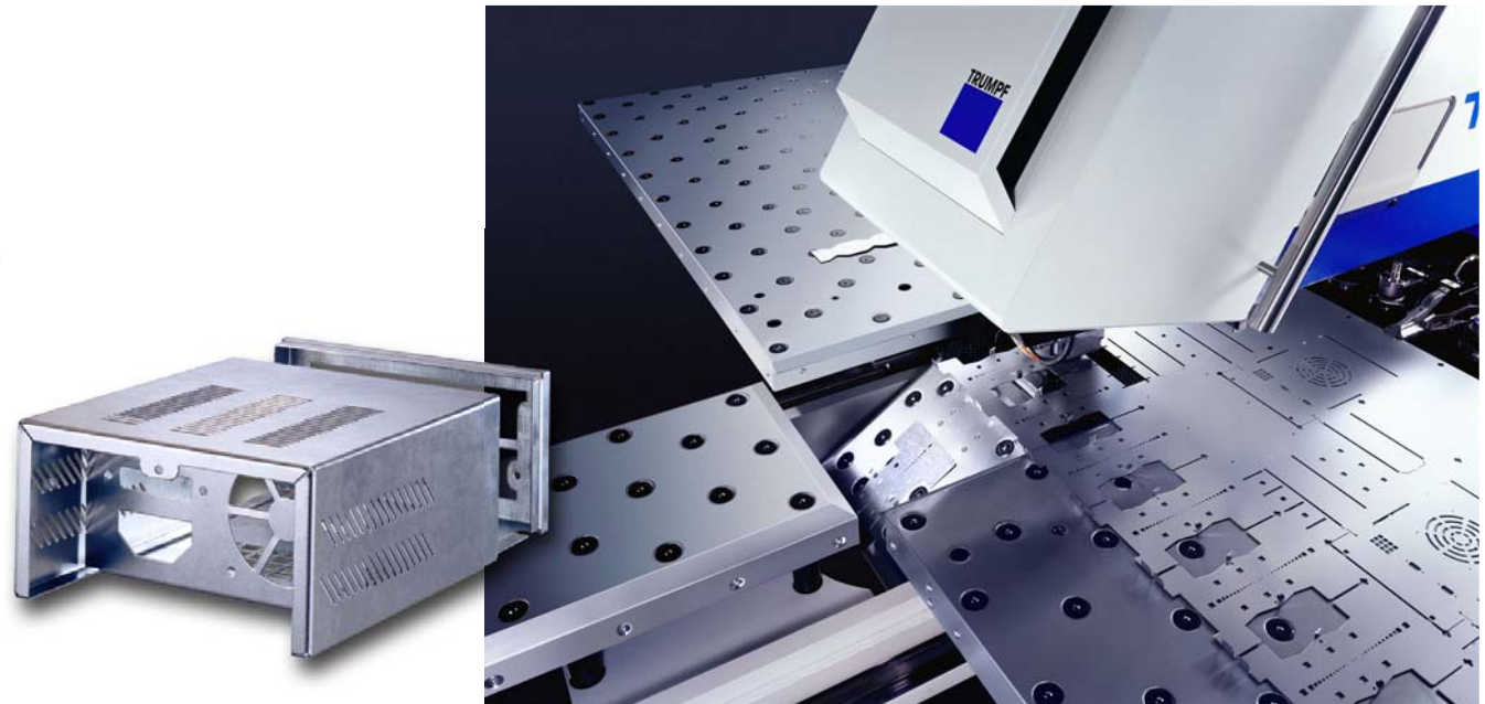
Le centre de poinçonnage automatisé Trupunch 3000 Le chargement des tôles est automatique ainsi que le déchargement des pièces triées.
